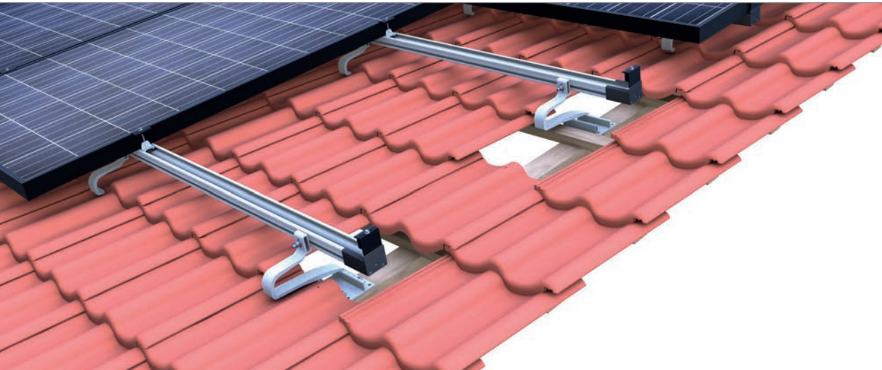
novotegra side-fix – Klemmsystem einlagig mit hochkant montierten Modulen
